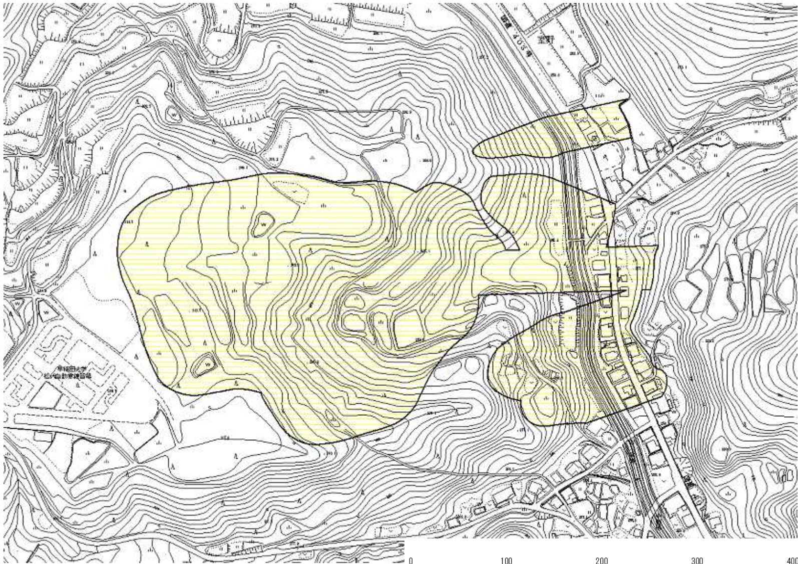
様式-2 (地) 土砂災害警戒区域 区域図
