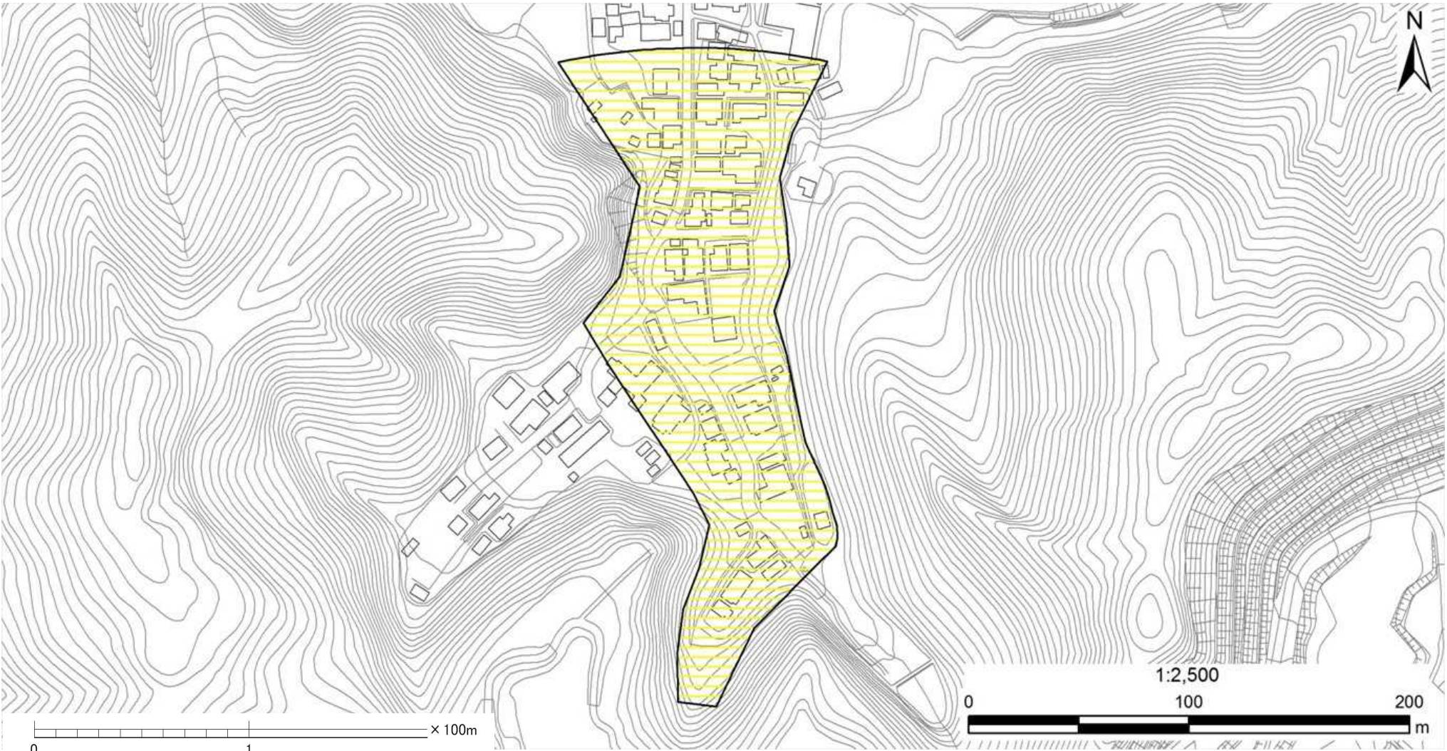
様式－２(土) 土砂災害警戒区域 区域図
